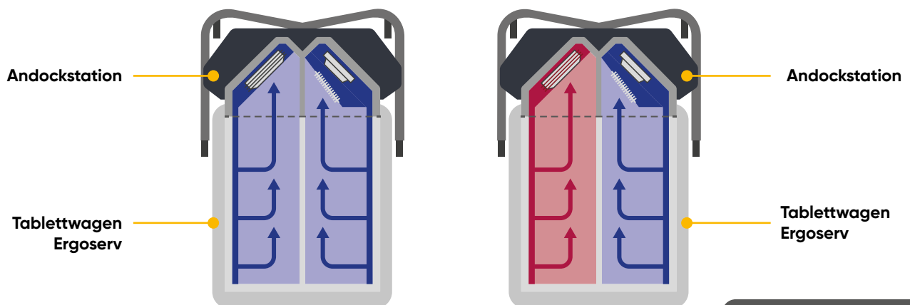
Draufsicht – Vertikalschnitt
